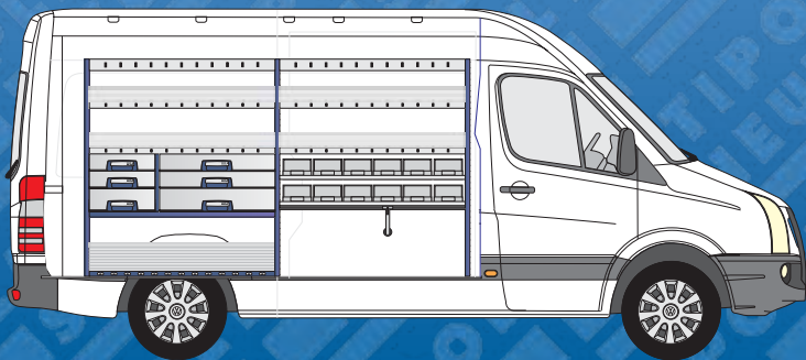
FAHRERSEITE (LINKS)
