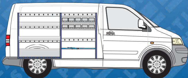
FAHRERSEITE (LINKS)
